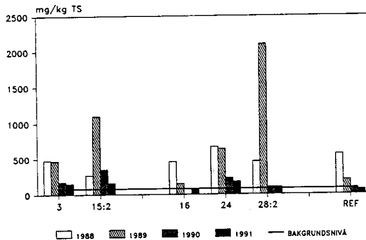
Figur 24. Innehållet av zink (mg/kg TS) i vattenmossa (Fontinalis) som varit utplanterad i ca 4 veckor på olika lokaler i Saxån -Braåns vattensystem 1991. REF = metallinnehållet i mossan före utplanteringen.
