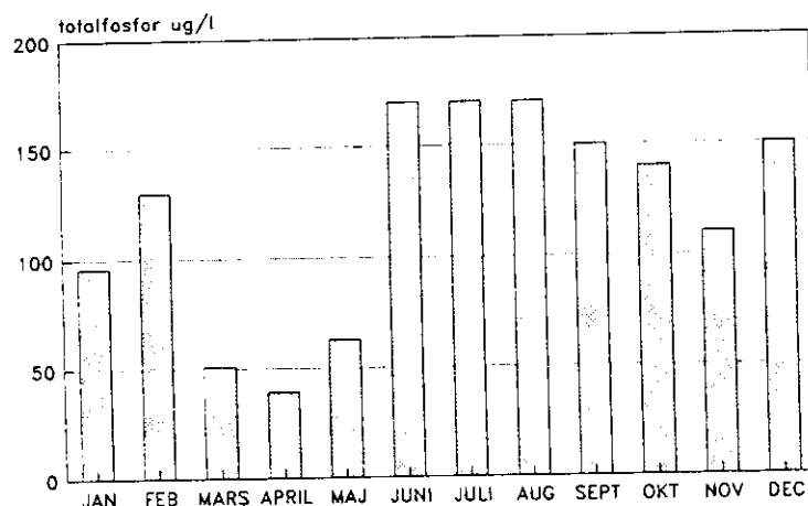
Figur 13. Totalfosforhalterna i Saxån vid provpunkt 16 1991. (månadsprovtagningar)
