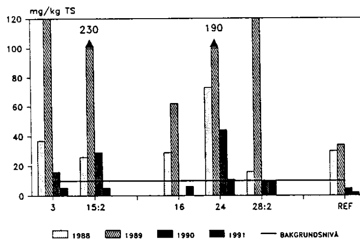
Figur 26. Innehållet av nickel (mg/kg TS) i vattenmossa (Fontinalis) som varit utplanterad i ca 4 veckor på olika lokaler i Saxån -Braåns vattensystem 1991. REF = metallinnehållet i mossan före utplanteringen.
