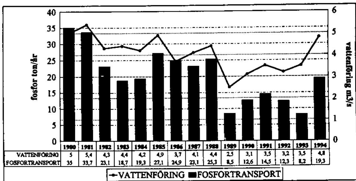
Figur 8. Totalfosfortransporten och årsmedelvattenföringen i Saxåns mynning under åren 1980 -1994.
